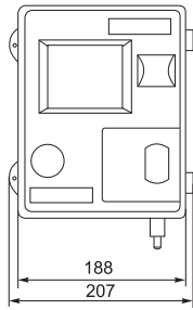
Габаритные и установочные размеры
