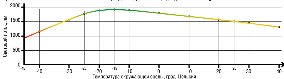
График зависимости светового потока от температуры окружающей среды для лампы Navigator NCL-SH10-28-E27/Outdoor
